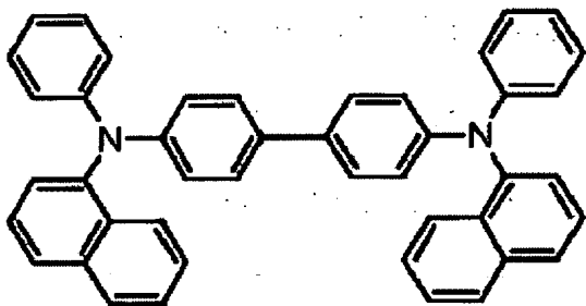
a-NPD:
